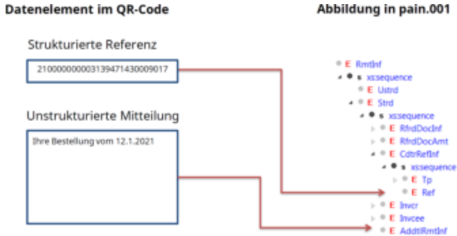
Abbildung 20: pain.001 – Verfahren mit strukturierter Referenz mit zusätzlichen Informationen
