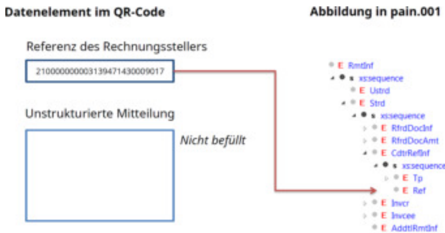
Abbildung 19: pain.001 – Verfahren mit strukturierter Referenz ohne zusätzliche Informationen
